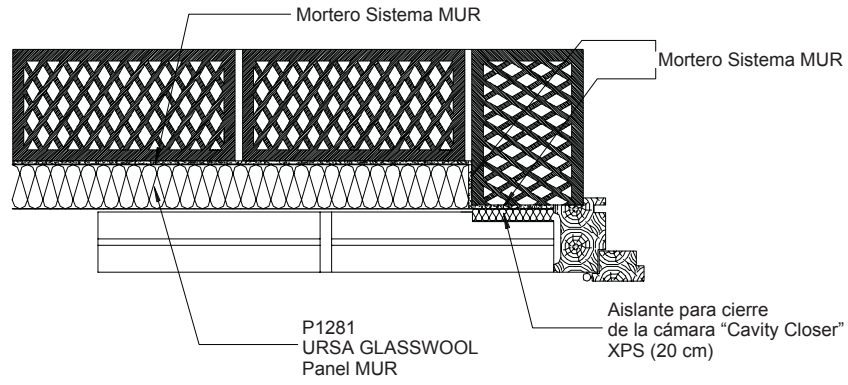
Figura 4. Jambas en ventana con corrección de puente térmico mediante "Cavity Closer".
