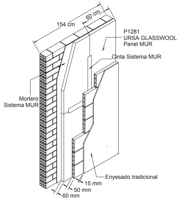
Figura 1. Configuración del Sistema URSA MUR.
