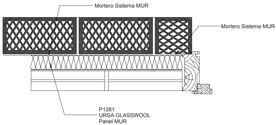
Figura 5. Jambas en ventana con corrección de puente térmico mediante carpintería.
